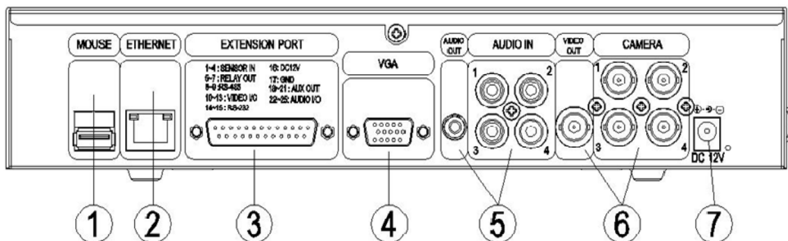
Illustration 2. Face arrière du DVR 4CH (4 canaux)
