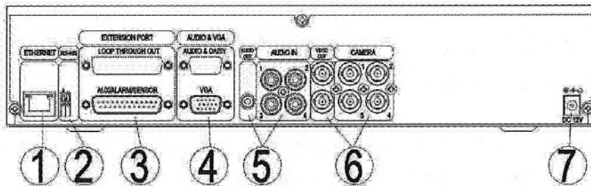
Illustration 2. Face arrière du DVR 4CH (4 canaux)
